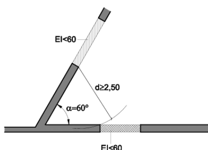
Figura 1.3. Fachadas a 60°
