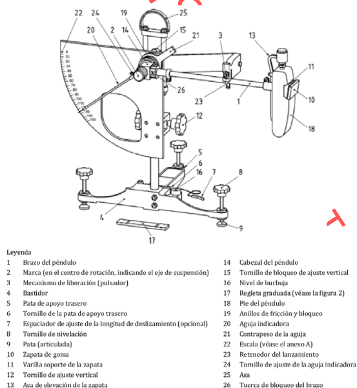
Figura 1. Péndulo de fricción
