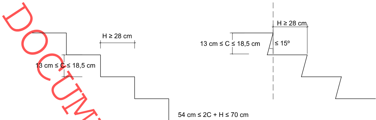
Figura 4.2 Configuración de los peldaños.
