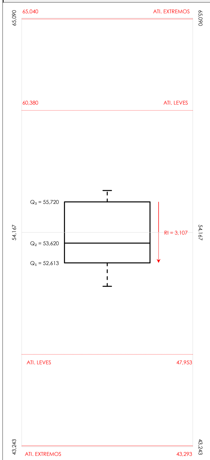
Diagrama Box-Plot post-estadístico. Eje Y: Int impactos estand fr3150 hz (DB)
