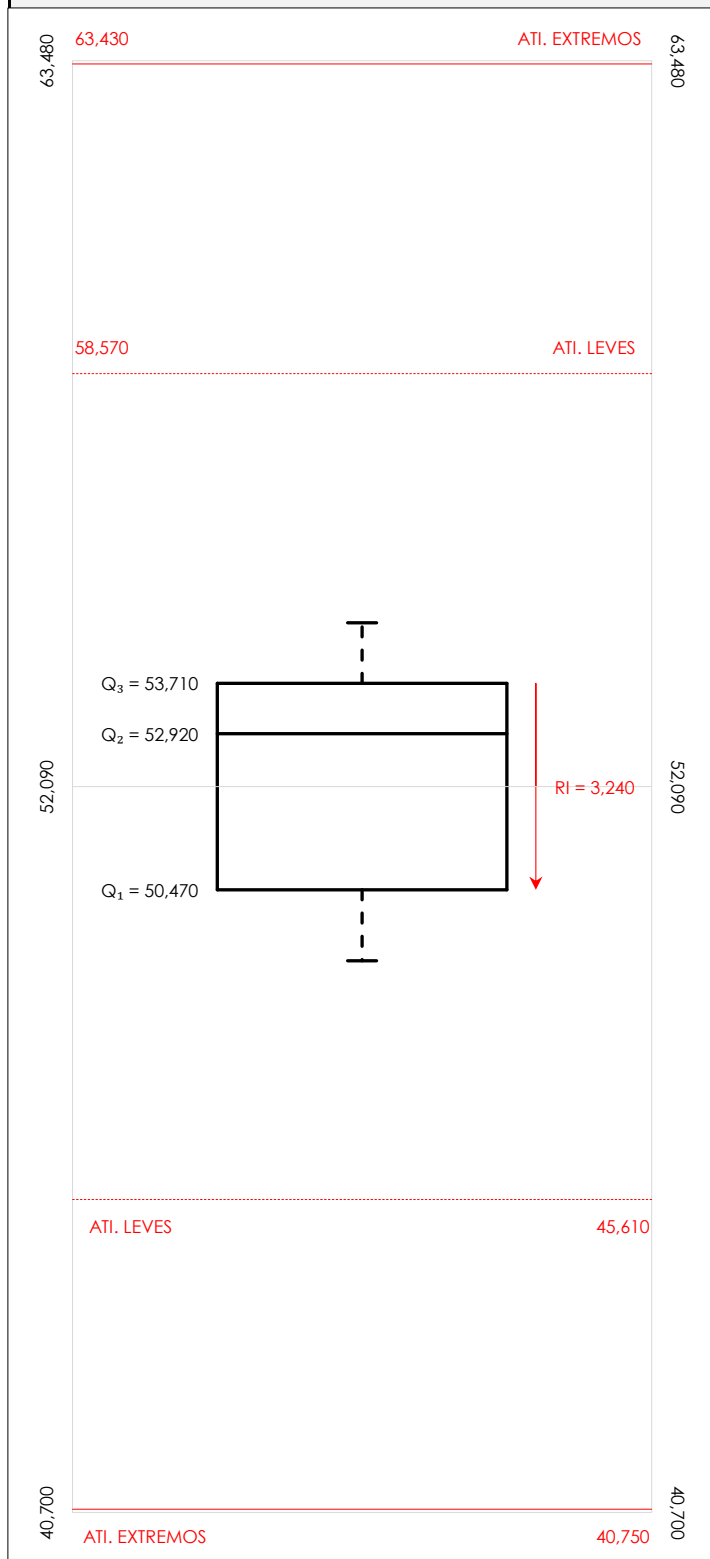
Diagrama Box-Plot post-estadístico. Eje Y: Int impactos estand fr4000 hz (DB)
