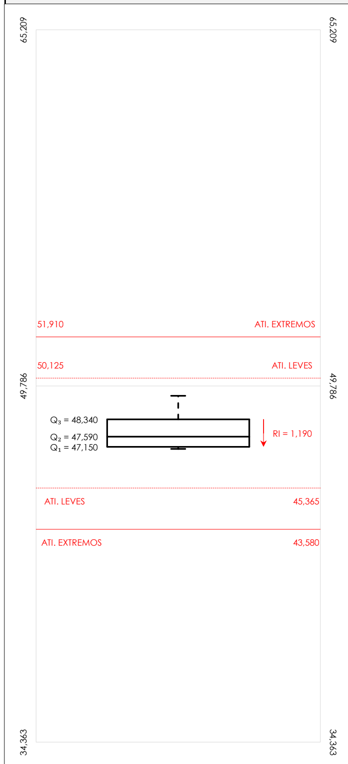
Diagrama Box-Plot post-estadístico. Eje Y: Int impactos estand fr250 hz (DB)
