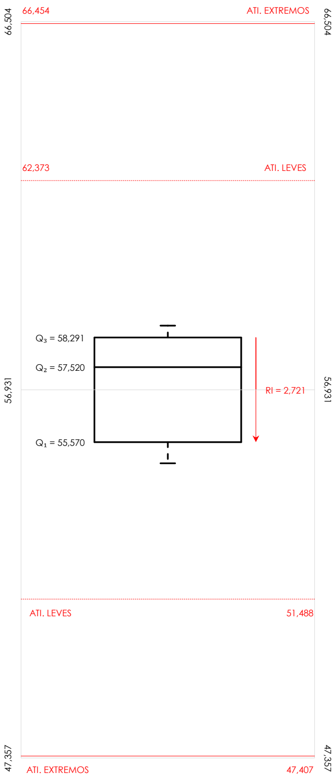
Diagrama Box-Plot post-estadístico. Eje Y: Int impactos estand fr1600 hz (DB)
