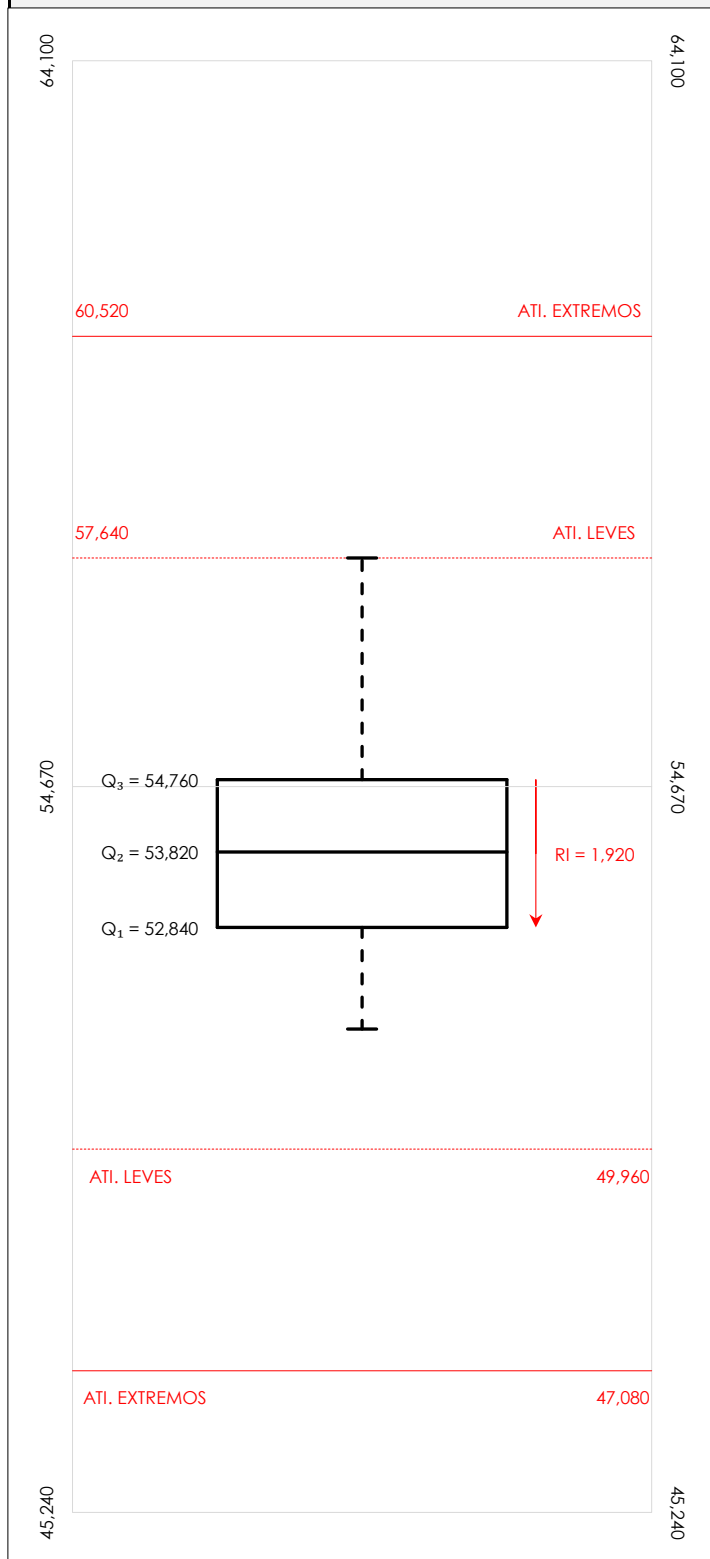
Diagrama Box-Plot post-estadístico. Eje Y: Int impactos estand fr1000 hz (DB)
