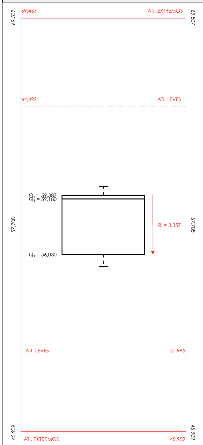
Diagrama Box-Plot pre-estadístico. Eje Y: Int impactos estand fr2000 hz (DB)
