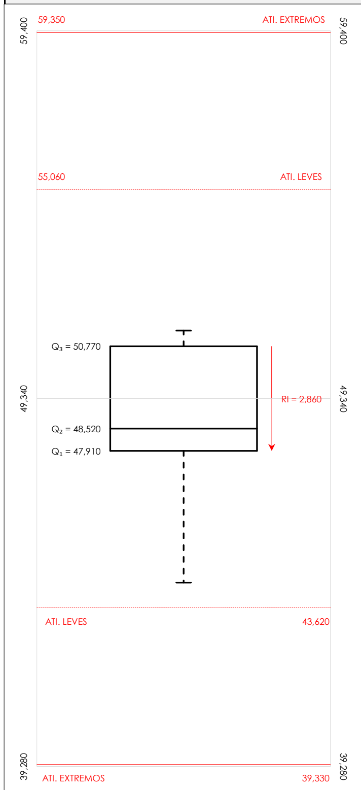
Diagrama Box-Plot pre-estadístico. Eje Y: Int impactos estand fr5000 hz (DB)
