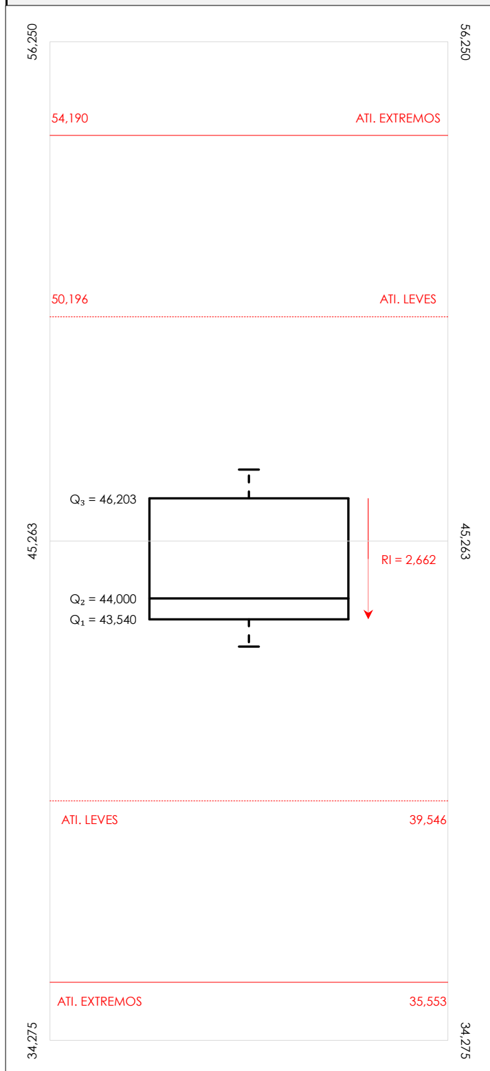
Diagrama Box-Plot pre-estadístico. Eje Y: Int impactos estand fr125 hz (DB)
