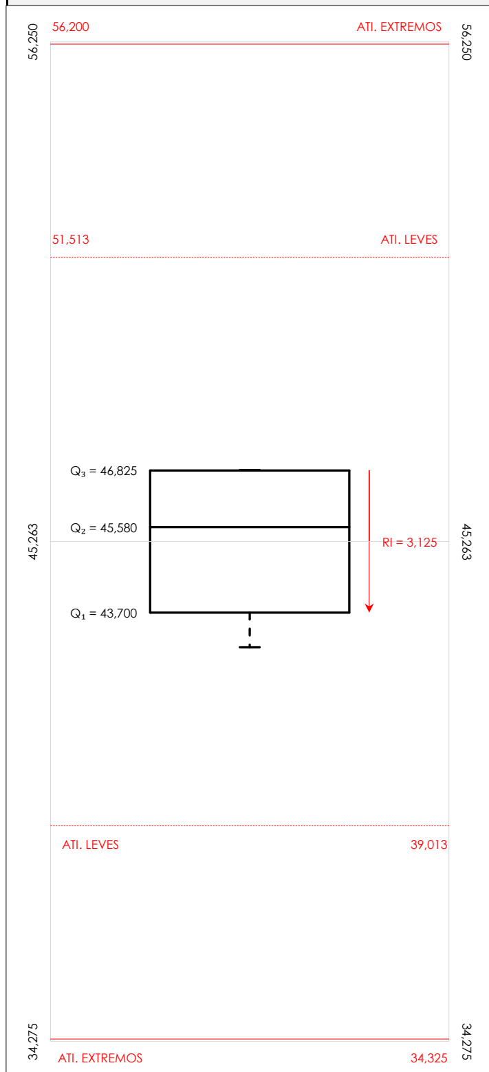
Diagrama Box-Plot post-estadístico. Eje Y: Int impactos estand fr125 hz (DB)
