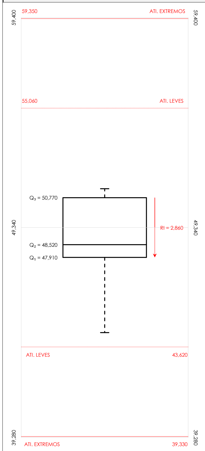
Diagrama Box-Plot post-estadístico. Eje Y: Int impactos estand fr5000 hz (DB)
