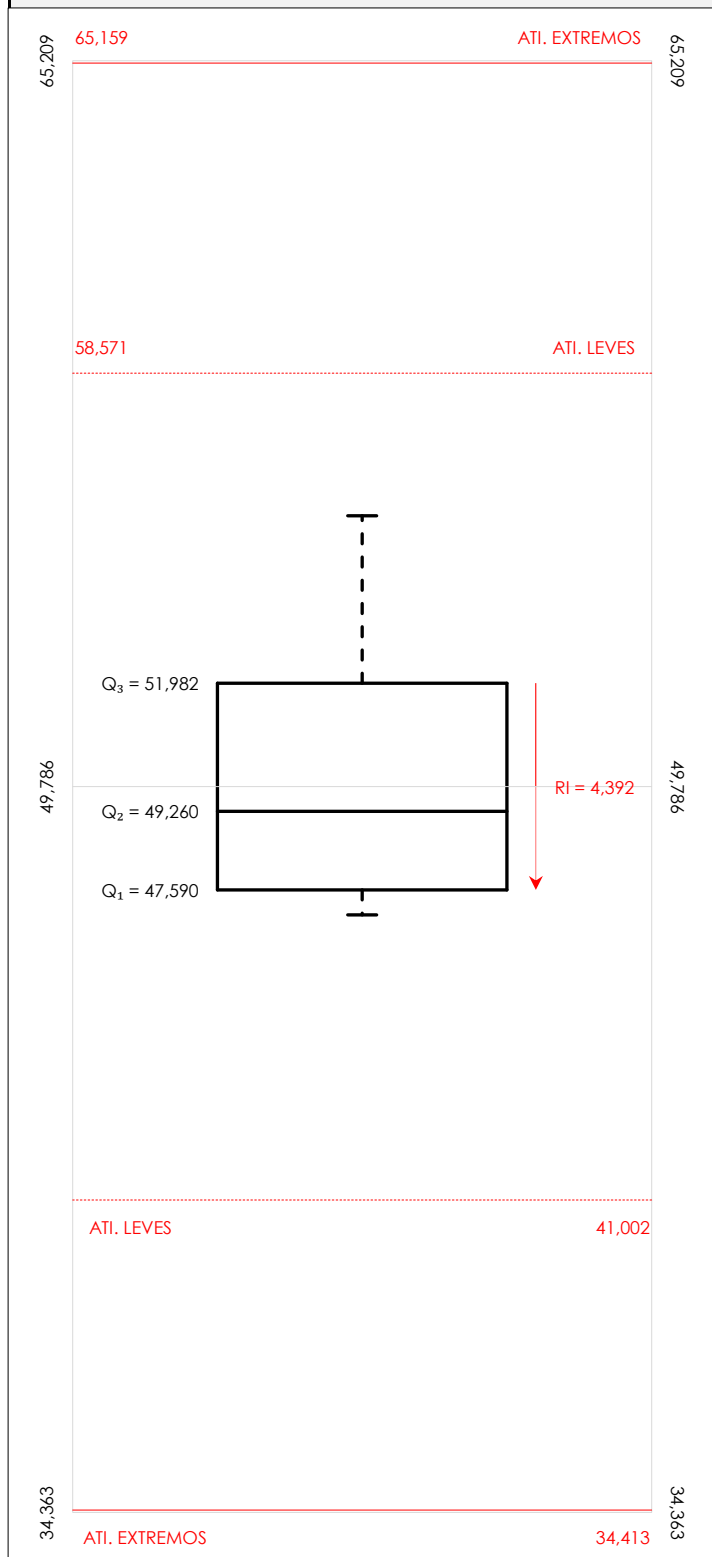
Diagrama Box-Plot pre-estadístico. Eje Y: Int impactos estand fr250 hz (DB)
