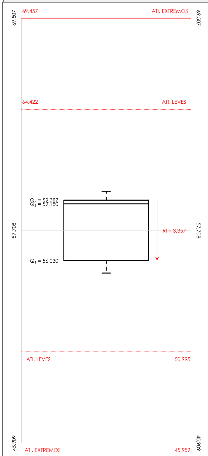
Diagrama Box-Plot post-estadístico. Eje Y: Int impactos estand fr2000 hz (DB)
