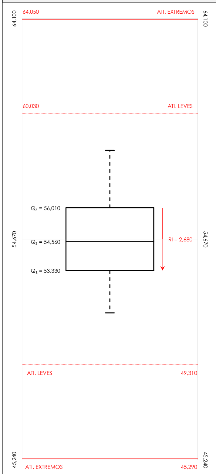
Diagrama Box-Plot pre-estadístico. Eje Y: Int impactos estand fr1000 hz (DB)
