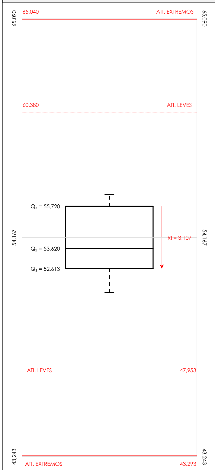
Diagrama Box-Plot pre-estadístico. Eje Y: Int impactos estand fr3150 hz (DB)
